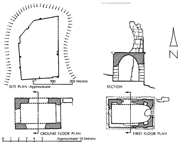
Ил. 2. План Сирменского монастыря, план северных ворот, поперечный разрез северных ворот и храма, план по уровню северной надвратной церкви.
