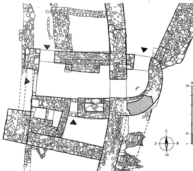
Ил. 8. Фуна. Надвратный храм и внешняя стена крепости. План.
