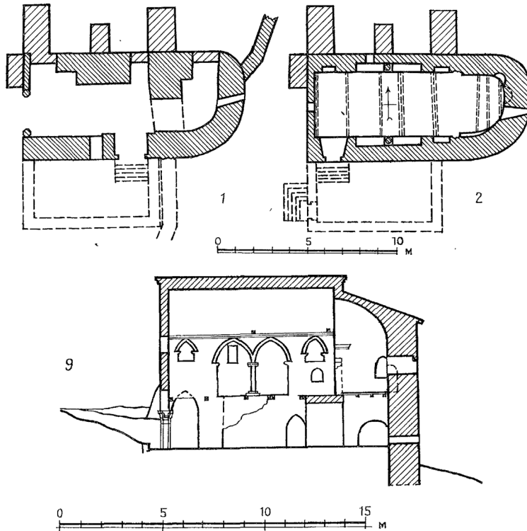
Ил. 7. Ворота и надвратный храм крепости Фуна. План нижнего и верхнего этажей; продольный разрез. Источник: Кирилко 1989, 65, 68.
